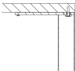
Verborgen centrale bevestiging van poot aan tafelblad.
